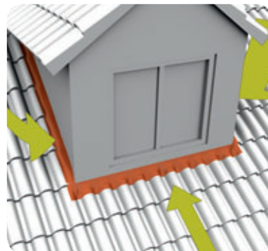
Handwerksgerechter Anschluss an Gauben.
