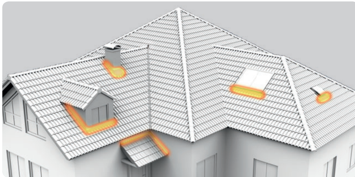
Wakaflex: vielseitig einsetzbar für Wand, Kamin, aufgehende Bauteile und andere Anschlüsse.
